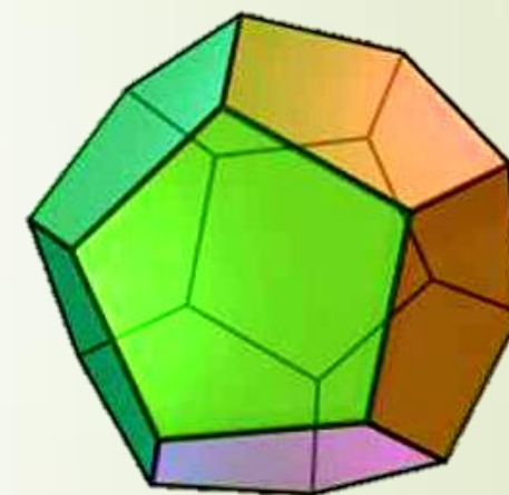
Додекаэд
