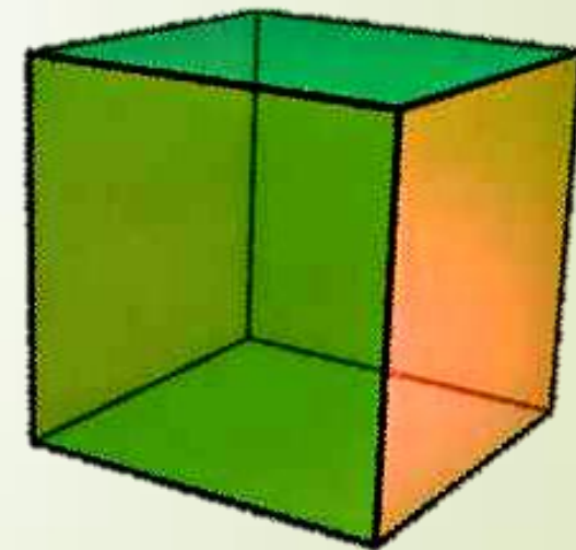
Куб (гексаэдр)
